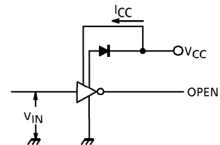
6. I_{CC}
