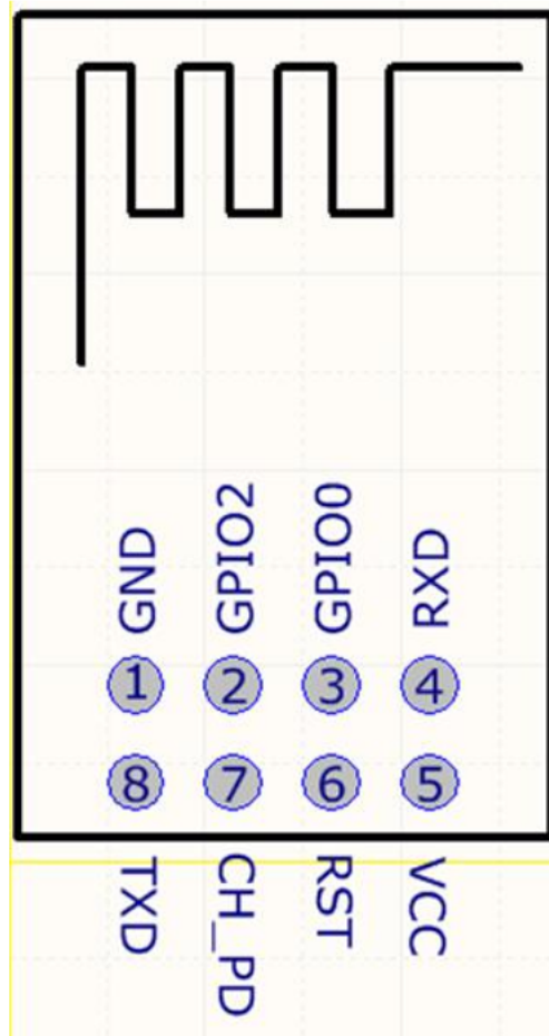
图 2 ESP-01S 管脚图
