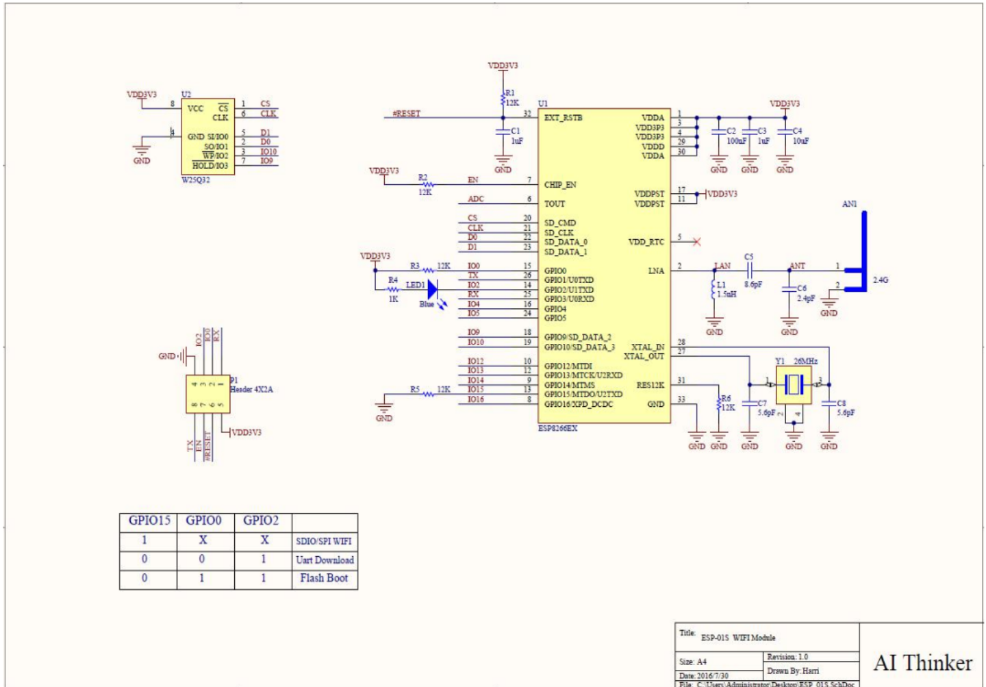
图 5 ESP-01S 原理图
